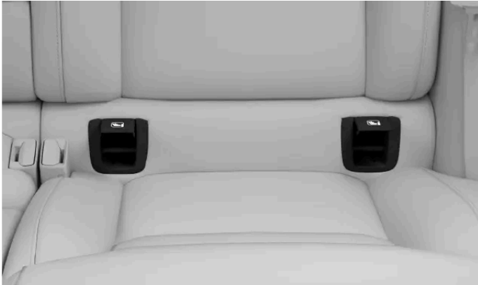
Locaties van ISOFIX-verankeringspunten voor de buitenste plekken van de achterbank
