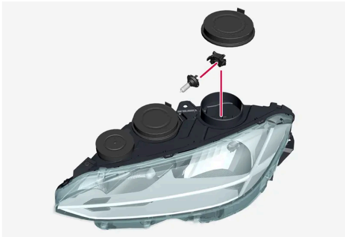
Linker koplamp.
