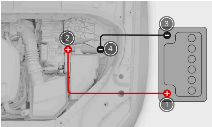
Aansluiting startkabels
