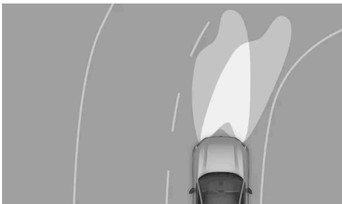
Funcionamento típico do farol autodirecional
