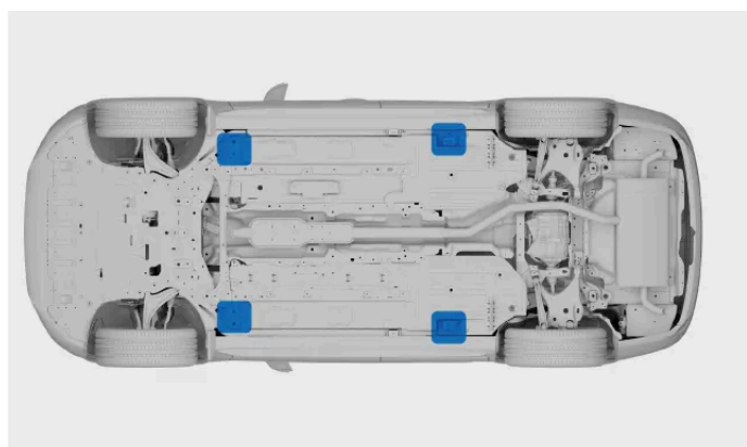
Áreas de elevação utilizadas para equipamentos de oficina.
