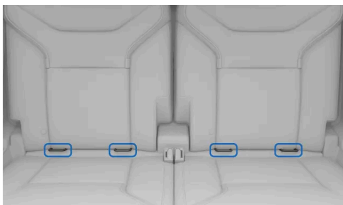
Emplacement des points d'ancrage ISOFIX [1] pour les sièges de la troisième rangée
