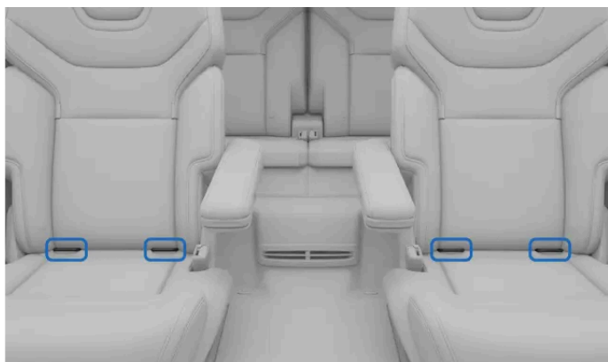
Emplacement des points d'ancrage ISOFIX [1] pour les sièges de la deuxième rangée
