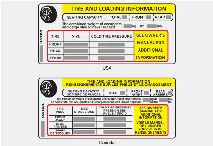
Étiquette de pression des pneus
