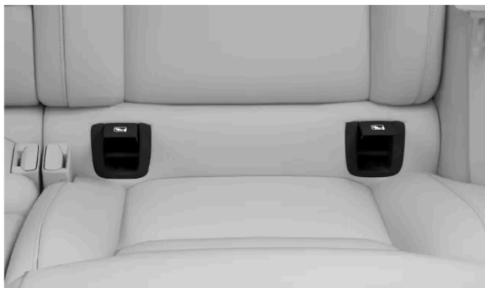
Umístění kotevních bodů ISOFIX na krajních zadních sedadlech
