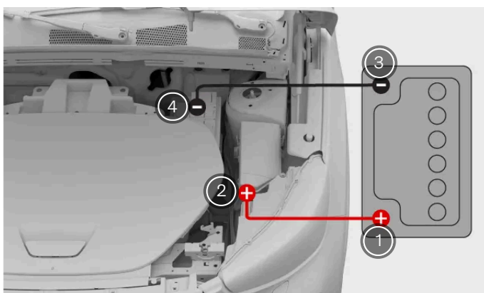
Starthilfekabel anschließen
