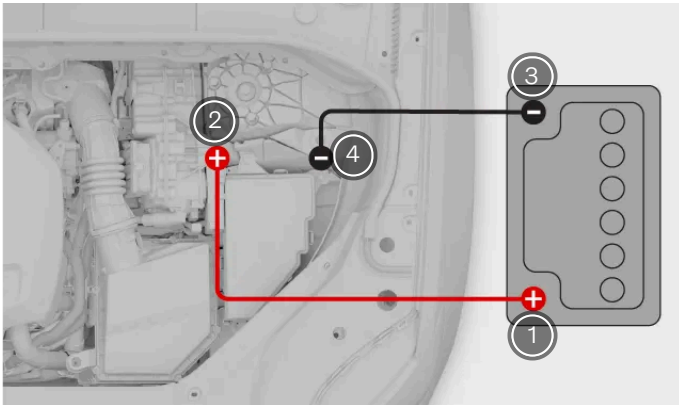
Starthilfekabel anschließen
