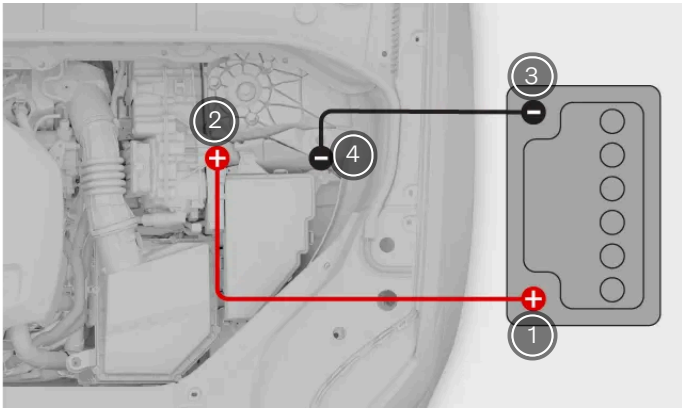
Starthilfekabel anschließen
