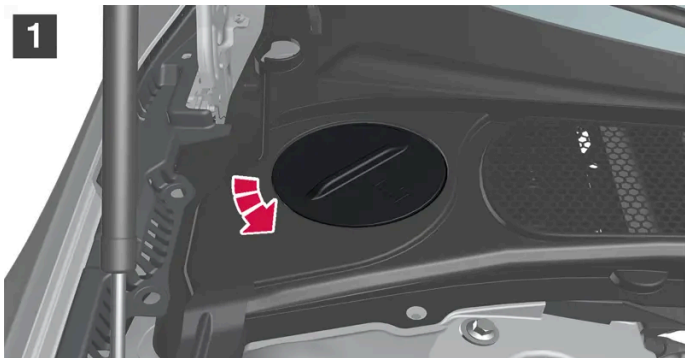
Ausgleichsbehälter der Kühlanlage, Linksenker.
