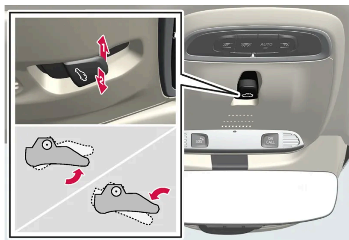
Ventilationsstilling, vertikalt bagtil.
