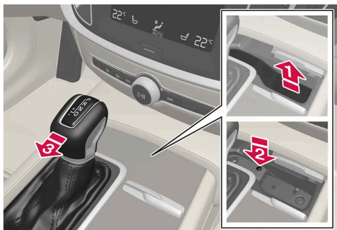
Oversigt over stor gearstang.
