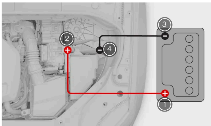
Käynnistyskaapeli kytkeä
