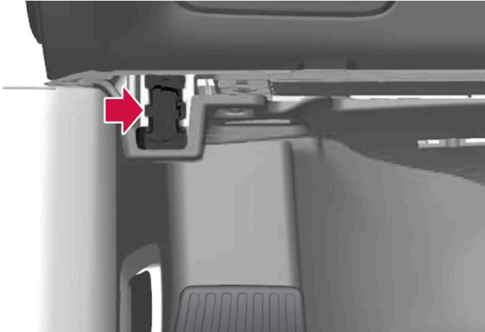
Diagnoosiulosotto (On-board Diagnostic -liitäntä, OBDII) kojelaudan alla kuljettajan puolella.
