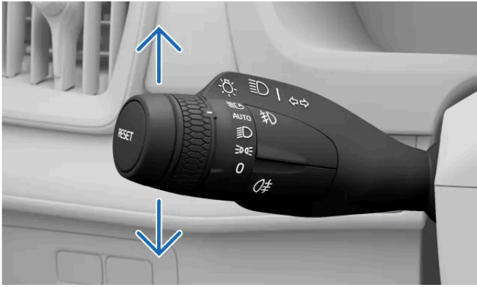
Suuntavilkujen säätimet vasemmanpuoleisessa vivussa
