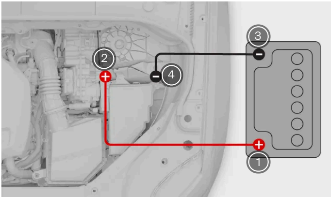
Käynnistyskaapeli kytkentä
