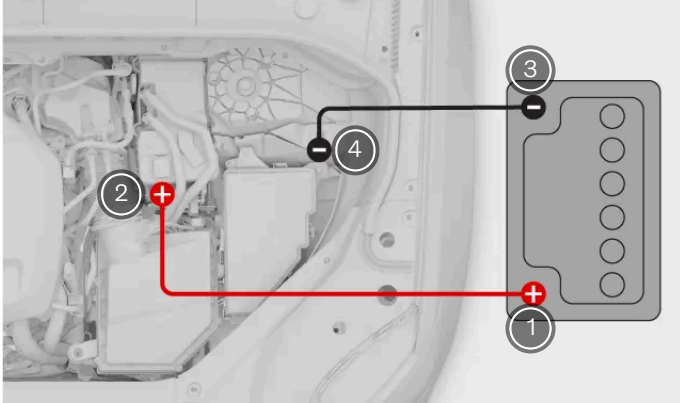
Käynnistyskaapeliin kytkeä
