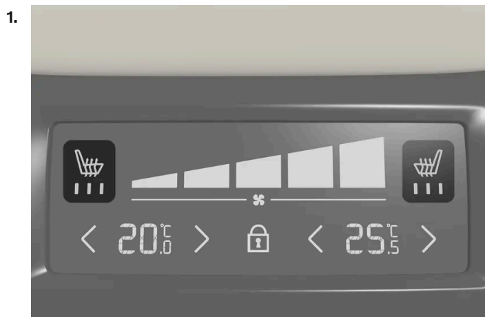
Témoin de siège chauffant et panneau de commandes climatiques arrière, sur la console de tunnel.
