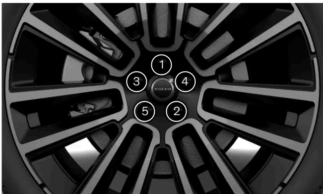
Σφίξτε τα μπουλόνια του τροχού χιαστί.
