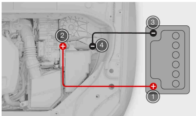
Σύνδεση καλωδίου βοηθητικής εκκίνησης
