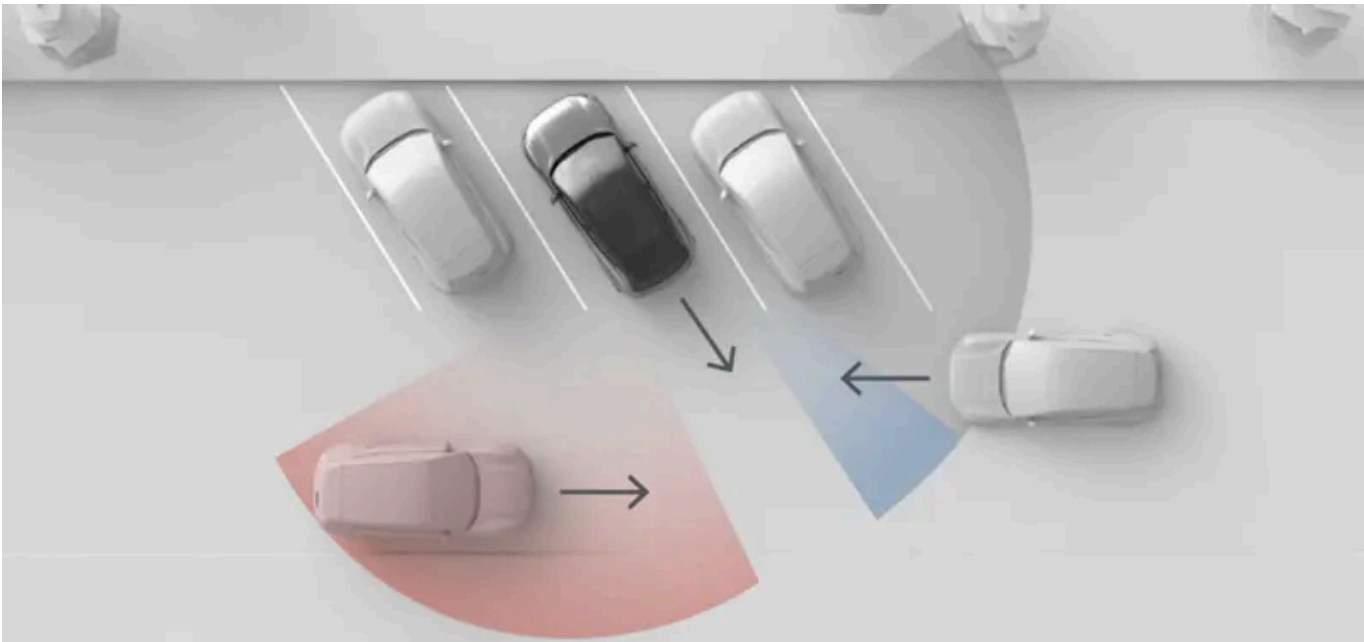
이 이미지에 표시된 상황은 주차된 차량과 같은 주변 물체가 레이더의 시야를 어떻게 제한할 수 있는지 보여줍니다. 장애물이 없는 상황에서는 유효 감지 영역이 양 쪽에서 동일합니다.
