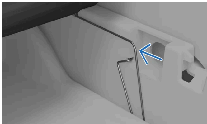
Rechter vergrendelingsclip.
