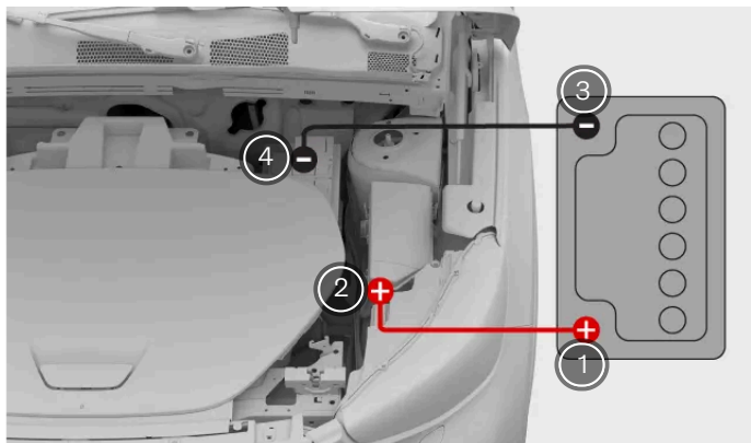
Aansluiting startkabels
