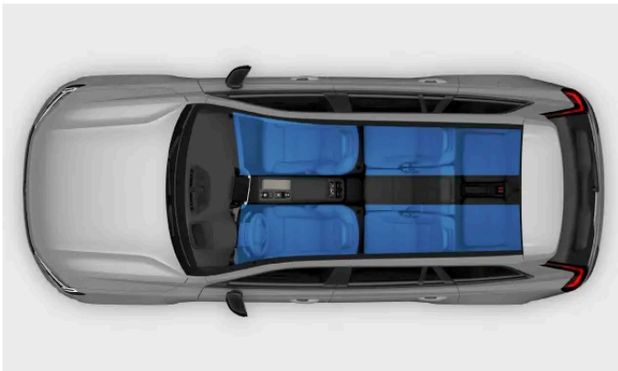
Klimaatzones
