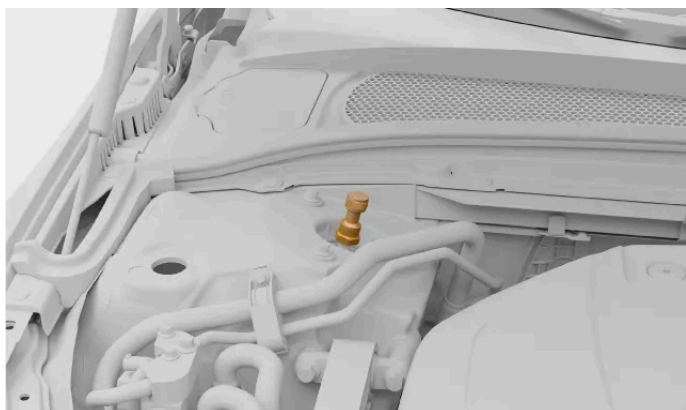
Pokrętła regulacyjne zawieszenia kół przednich znajdują się pod maską.
