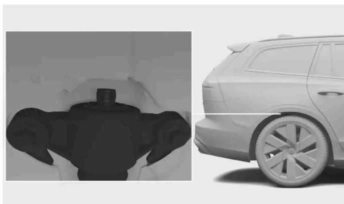
Pokrętło regulacyjne zawieszenia kół tylnych znajduje się nad każdym kołem tylnym, w jego wnętrzu.
