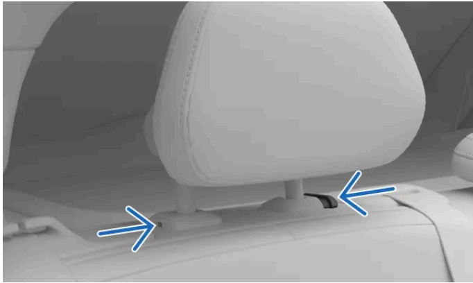
Butoanele utilizate pentru demontarea tetierelor.
