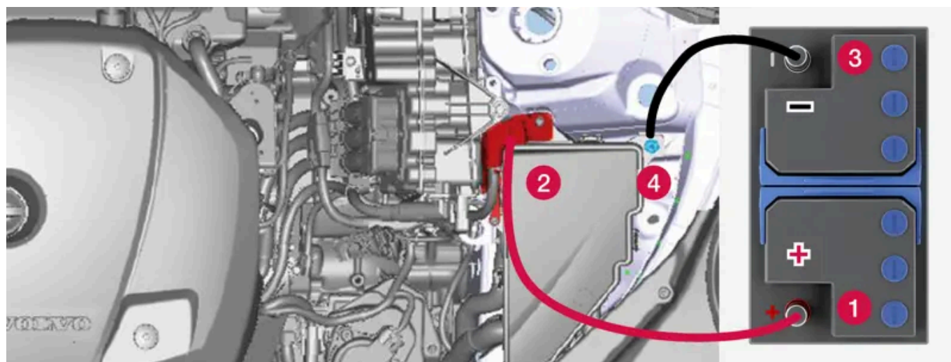
Punctele de încărcare pentru pornirea asistată a propriei mașini.
