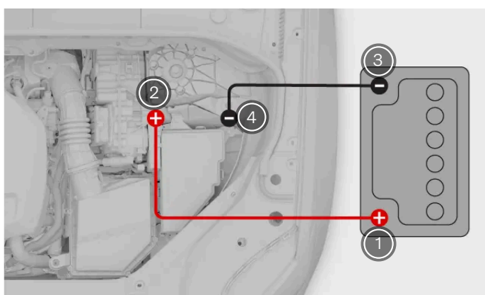
Anslutning av startkabel
