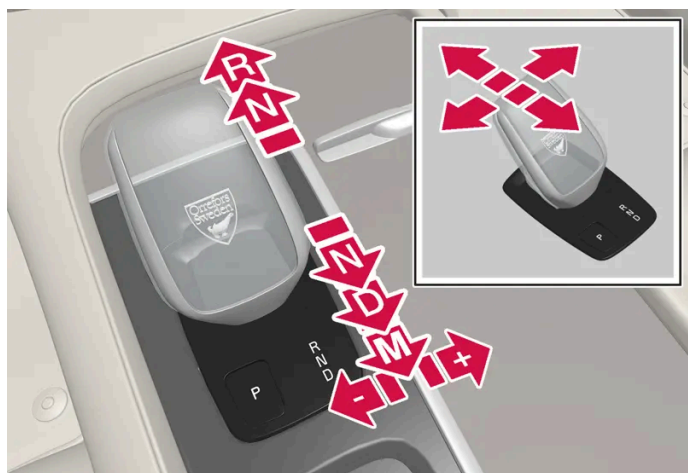
Visão geral da alavanca de marchas e posições das marchas.
