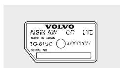
Etiqueta da caixa de câmbio
