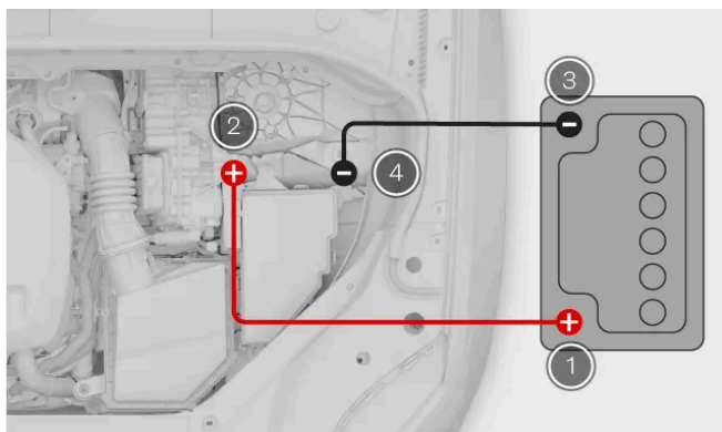
Connexion du câble de démarrage
