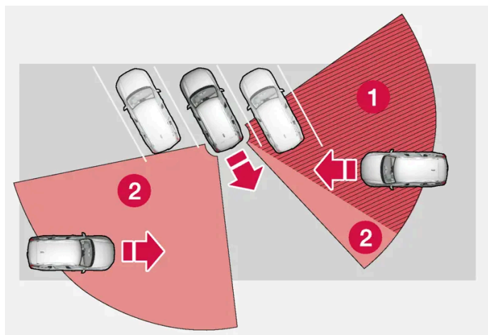
Je-li parkovací místo šikmé, systém Cross Traffic Alert může být na jedné straně zcela "slepý".
