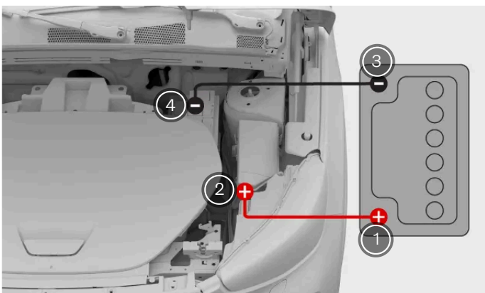
Starthilfekabel anschließen
