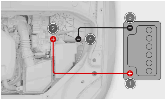
Starthilfekabel anschließen
