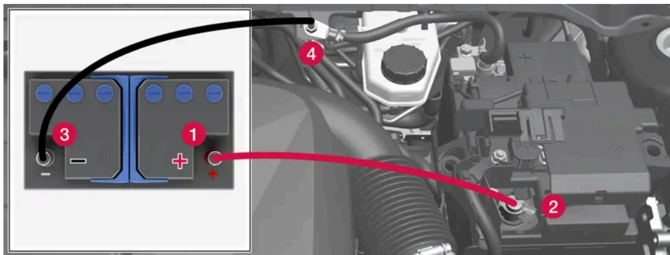
Puntos de fijación de los cables de arranque.
