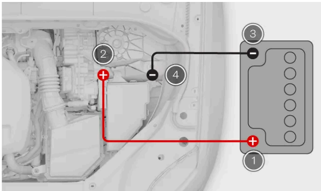
Conexión del cable puente
