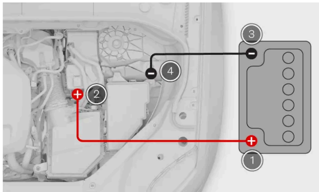
Käynnistyskaapeli kytkeä
