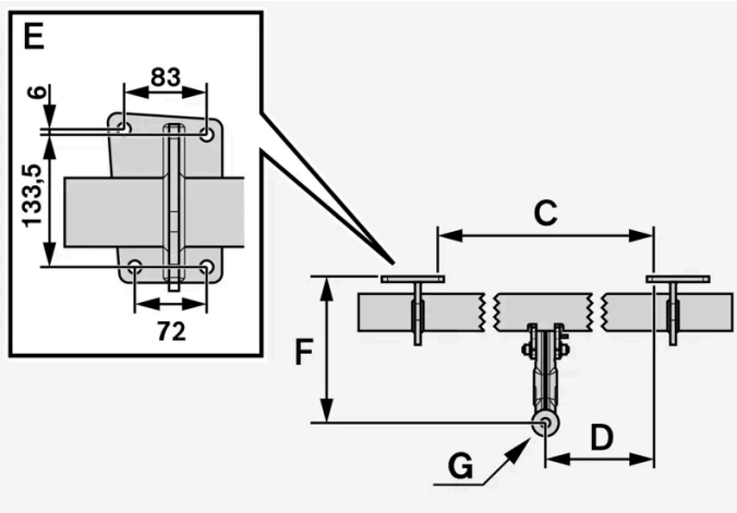
장착점 치수, mm (인치)
