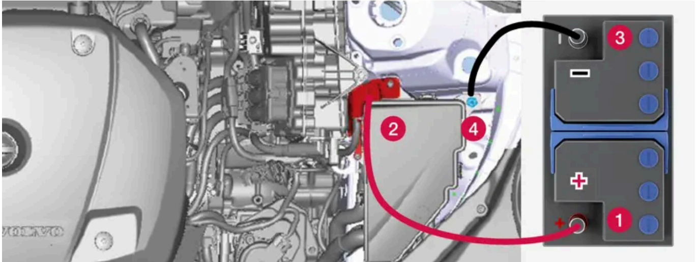
차량의 점프 시동 충전 포인트. 엔진룸의 외관은 차량 모델 및 옵션 레벨에 따라 다를 수 있습니다.
