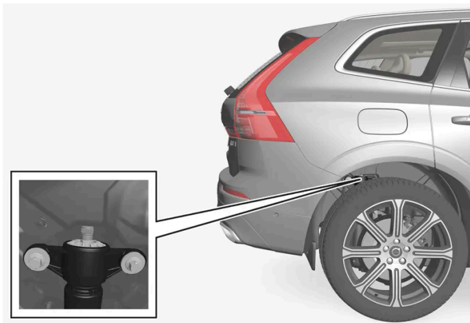
어저스터 노브의 위치, 뒷바퀴
