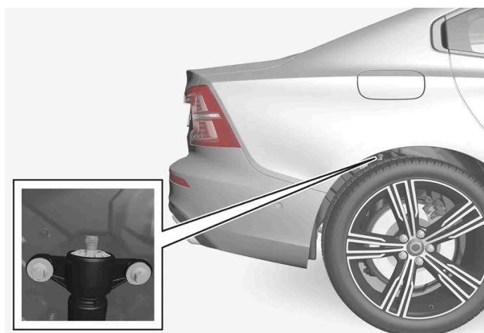
Plaatsing instelknop achterwiel.
