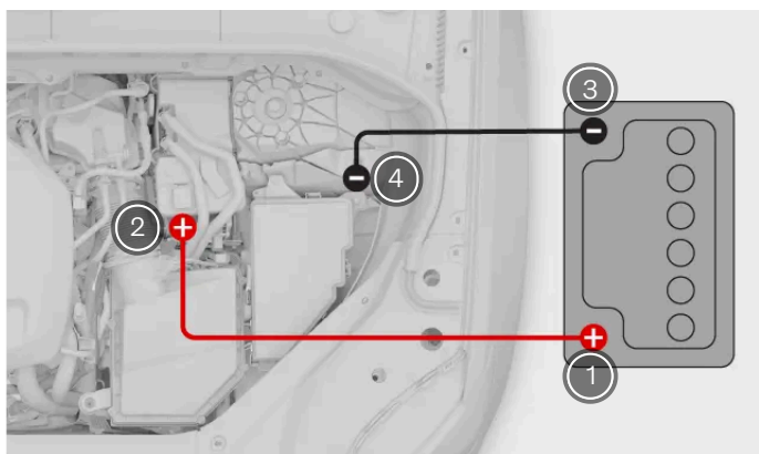
Aansluiting startkabels
