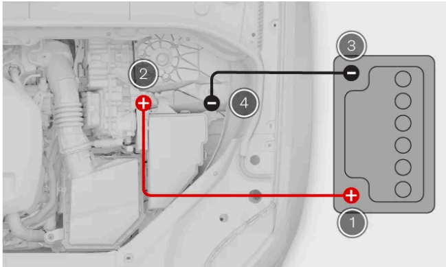
Aansluiting startkabels
