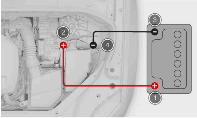
Tilkobling av bytteledning
