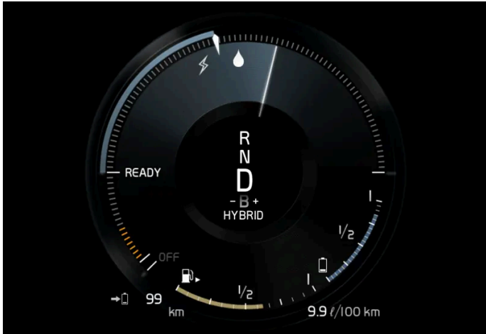
Førerdisplayet ved framdrift med både elektrisk motor og forbrenningsmotor.
