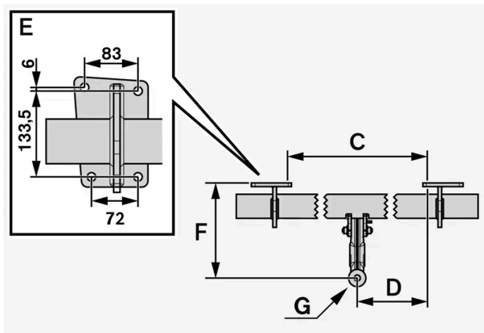
Mål, festepunkter i mm (tommer)
