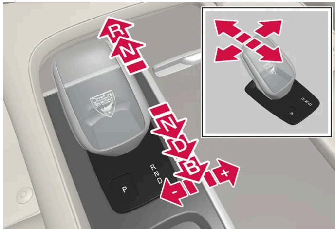
Prezentacja dźwigni zmiany biegów i układu biegów.
