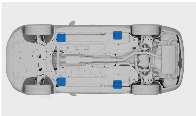
Lyftområden som används för verkstadsutrustning.
